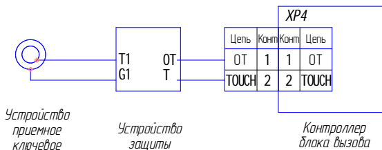
Схема подключения устройства защиты для блоков вызова ЦИФРАЛ CCD-2094.1, CCD-2094.1/V
