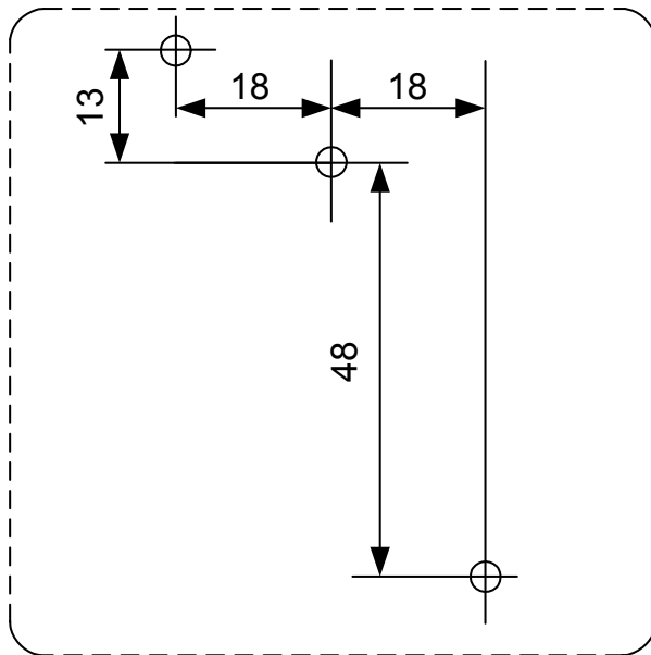
Рисунок 2. Разметка для крепления на стену
