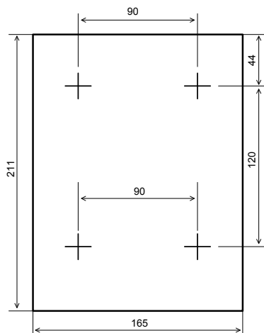
Рисунок 2. Габаритно-установочные размеры
