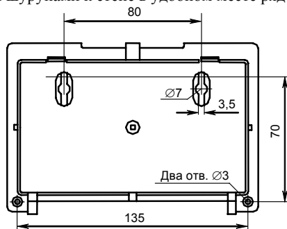
Рисунок 2 Габаритные и установочные размеры «С2000-USB»
