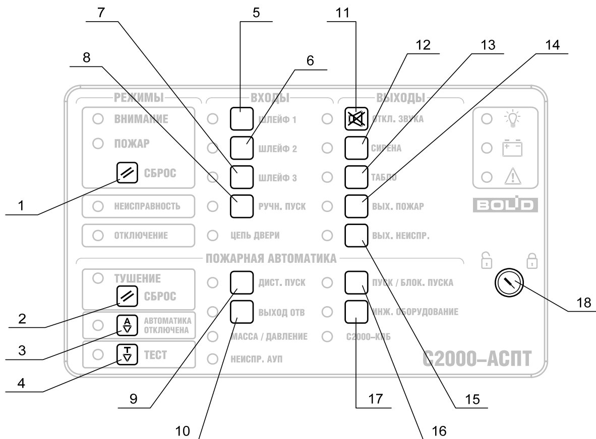
Рисунок 2.2 Расположение кнопок
