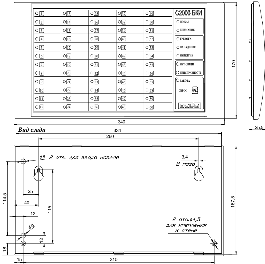
Рисунок 1. Внешний вид, габаритные и установочные размеры блока
