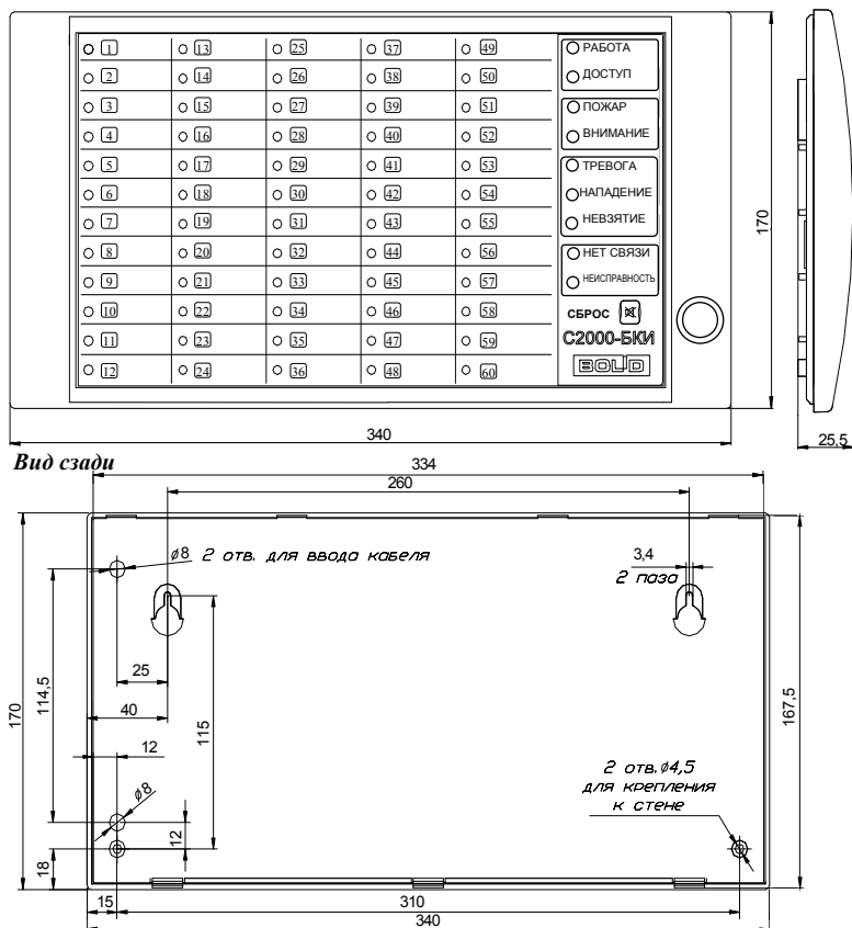
Рисунок 1. Внешний вид, габаритные и установочные размеры блока
