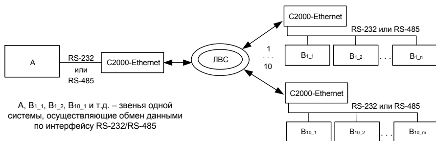
Рисунок 2 Общая схема использования «С2000-Ethernet» в «прозрачном режиме»
