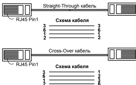
Рисунок 6 Типы Ethernet-кабелей
