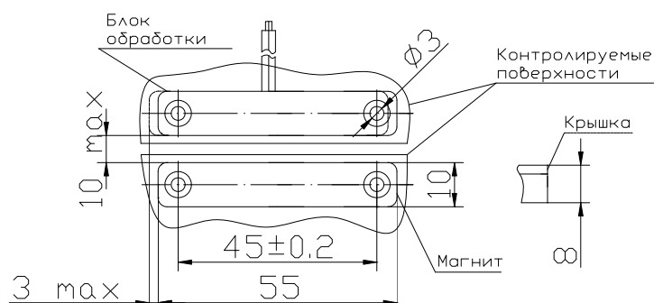
Рисунок 2 Установочные размеры
