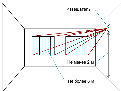
Рис. 3 Установка извещателя на боковой стене
