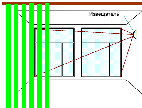
Рис. 6 Установка извещателя между стеклом и занавесками (жалюзи)
