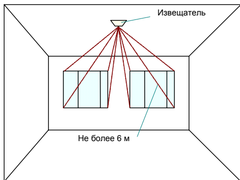
Рис. 2 Установка извещателя на потолке
