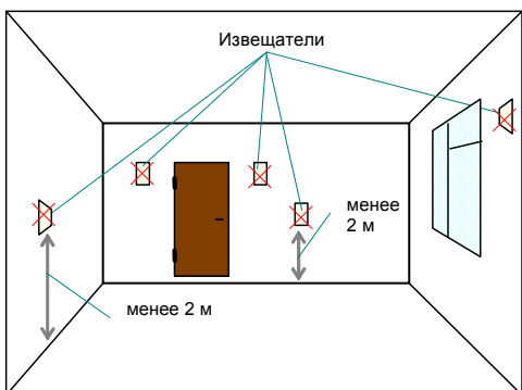
Рис. 7 НЕрекомендуемые места установки извещателя
