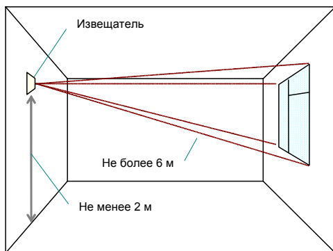
Рис. 4 Установка извещателя на противоположной стене
