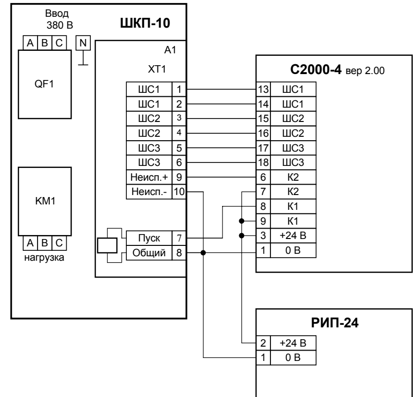
Рис 2 Пример подключения шкафа "ШКП-10" к прибору С2000-4
