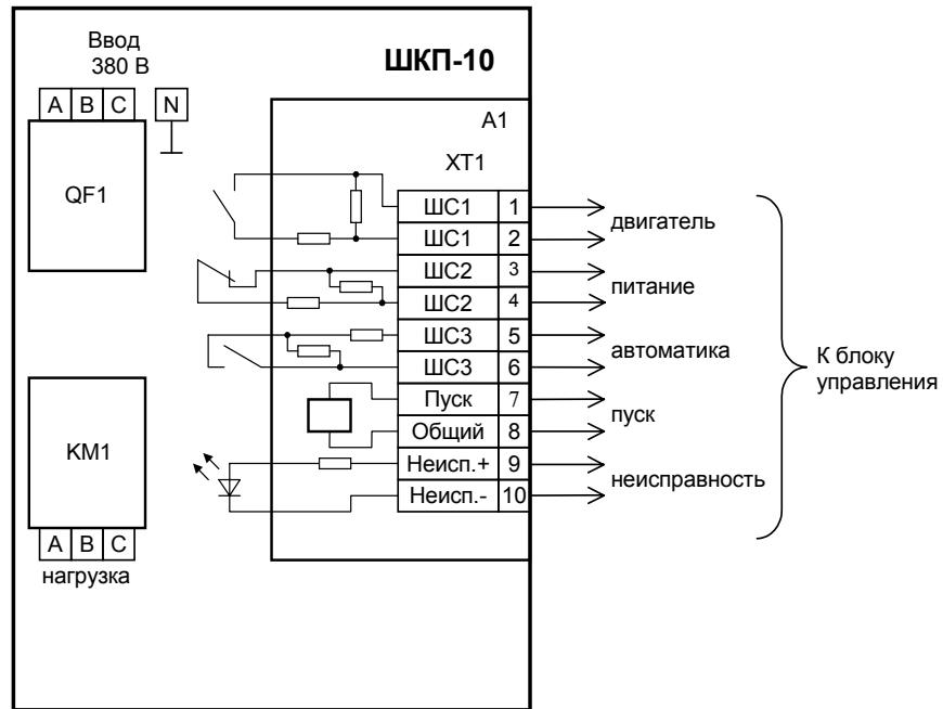
Рис 1 Схема электрическая подключения шкафа "ШКП-10" при эксплуатации
