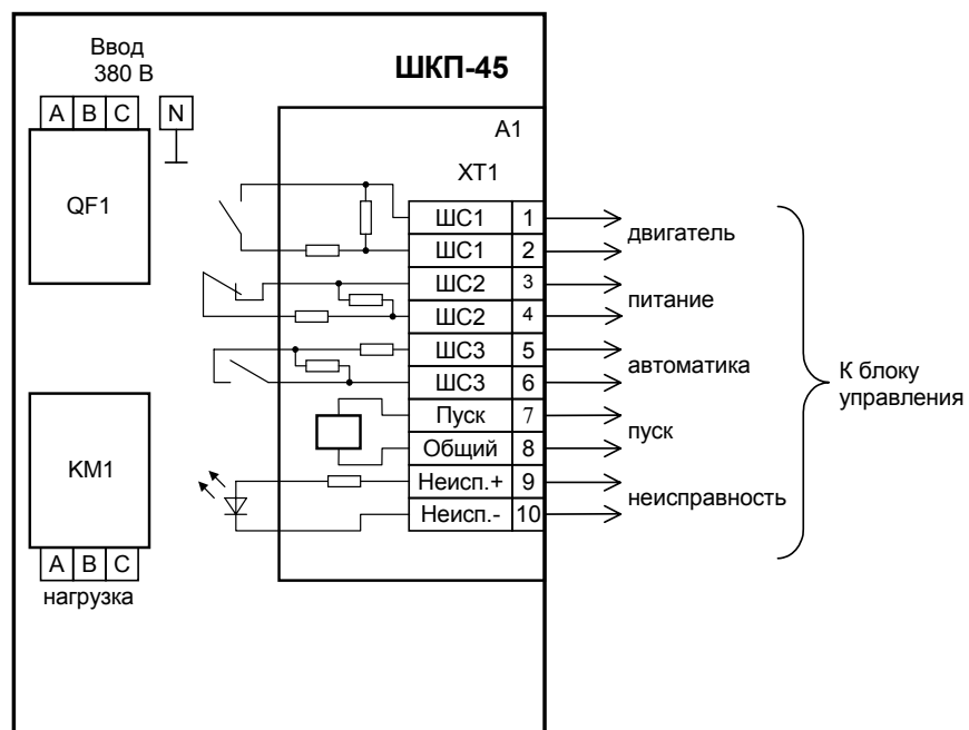
Рис 1 Схема электрическая подключения шкафа "ШКП-45" при эксплуатации
