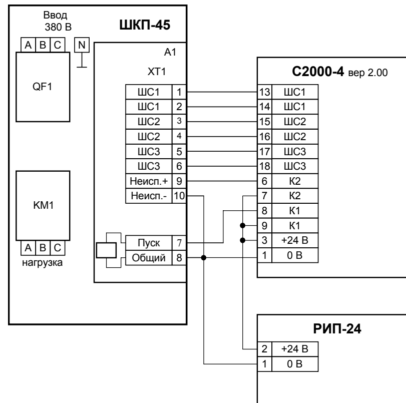
Рис. 2 Пример подключения шкафа "ШКП-45" к прибору С2000-4
