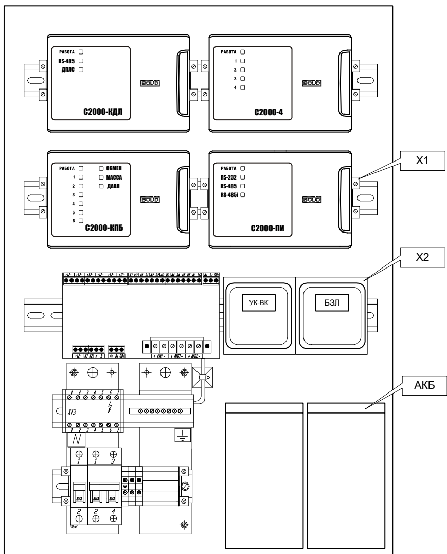
Рисунок 2 Пример компоновки «ШПС»
