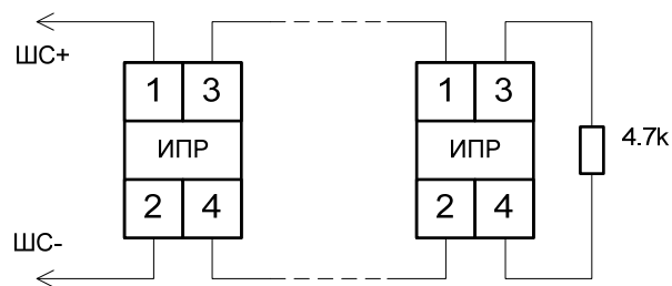
Подключение извещателей ИПР513-3
