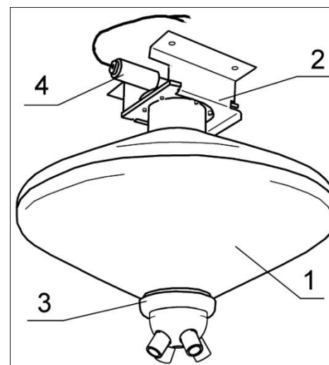
Рис. 1 – Конструкция МПП
