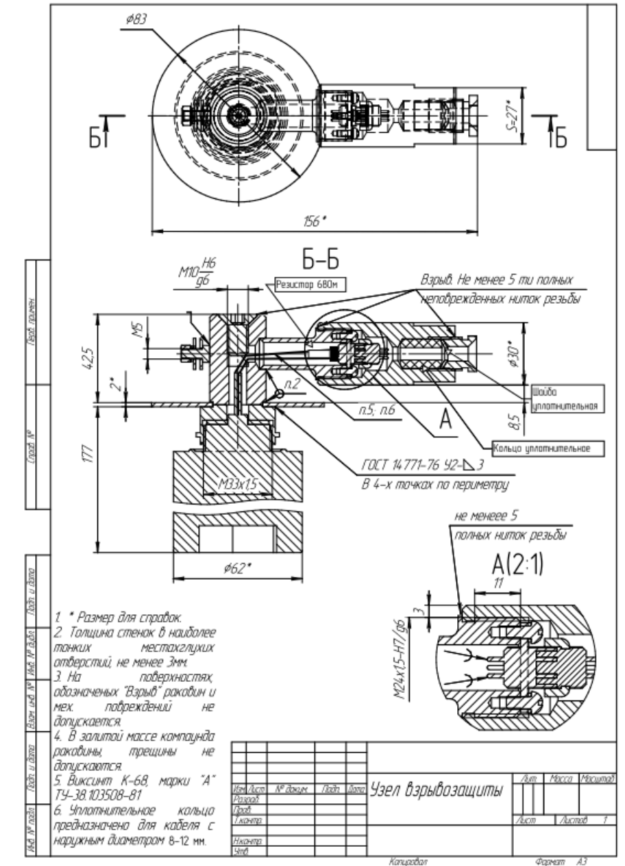
Рис. 2 — Чертёж средств взрывозащиты МПП
