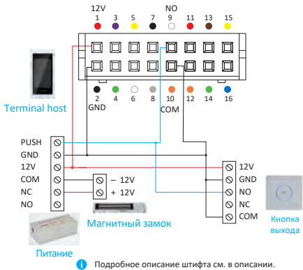
Схема установки системы для электромагнитной двери
