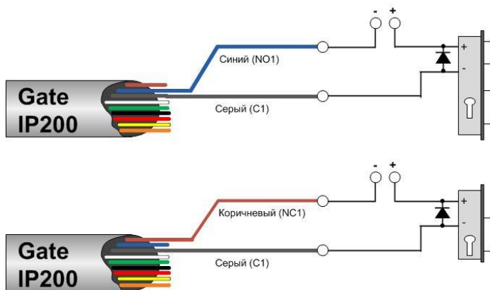
Рис.17. Подключение замков
