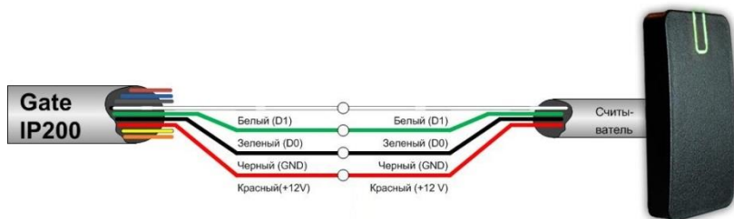
Рис.10. Подключение внешнего считывателя
