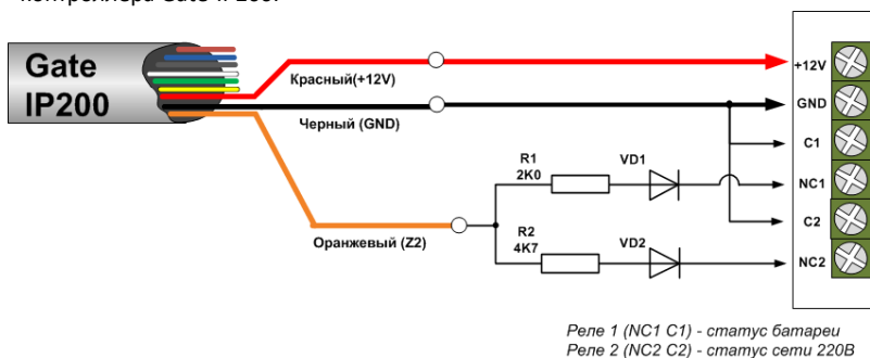
Рис.16. Подключение шлейфа контроля 220В и АКБ к PSU
