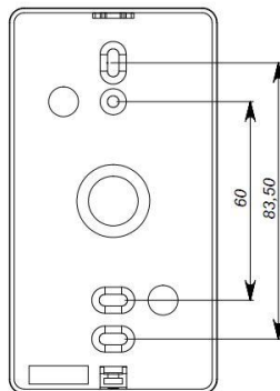
Рис. 8. Задняя пластина
