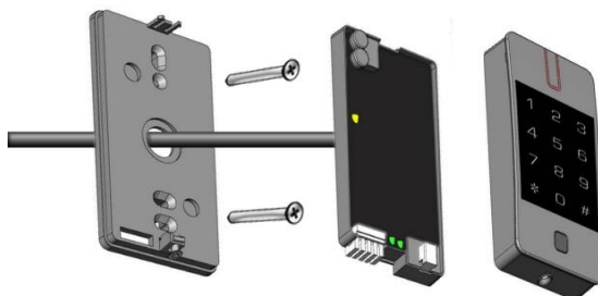
Рис. 9. Установка контроллера
