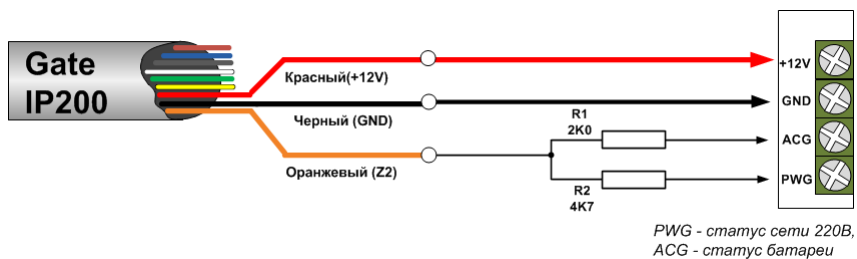
Рис.14. Подключение шлейфа контроля 220В и АКБ к PSU
