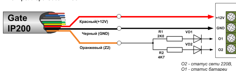
Рис.15. Подключение шлейфа контроля 220В и АКБ к PSU
