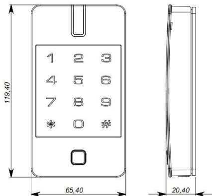
Рис 7. Габаритные размеры
