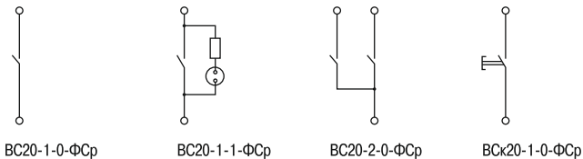
Рисунок 1 – Электрические схемы выключателей серии «ФОРС»
