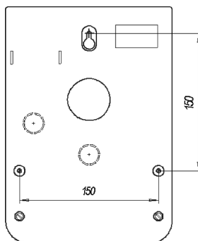
Рис. 2 Расположение отверстий для крепления на основании АС-2-3
