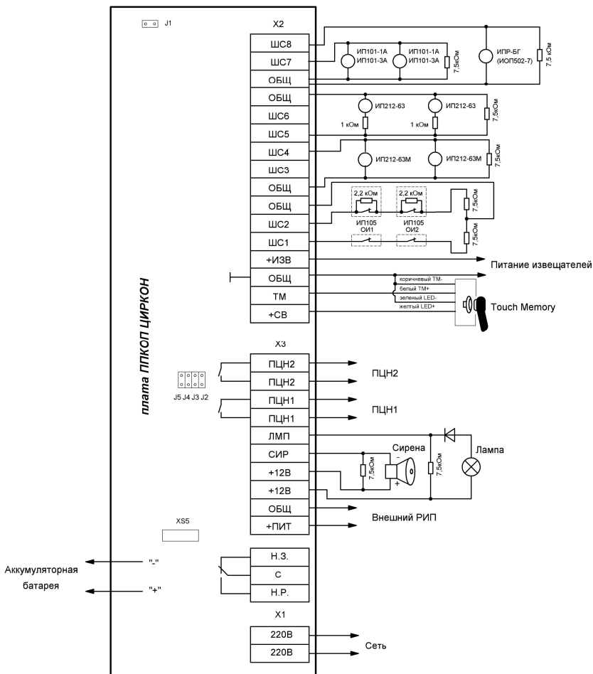
Рис. 3 Схема внешних соединений ППКОП «ЦИРКОН-8»
