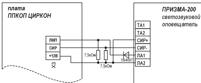
Рис. 5 Подключение светозвукового оповещателя «ПРИЗМА-200»
