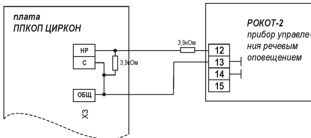
Рис. 7 Подключение прибора речевого оповещения «РОКОТ-2»
