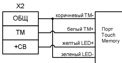
Рис. 2 Схема подключения порта Touch Memory к прибору
