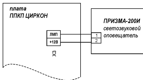
Рис. 4 Схема подключения светозвукового оповещателя «ПРИЗМА-200И»
