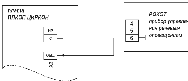
Рис. 6 Подключение прибора речевого оповещения «РОКОТ»
