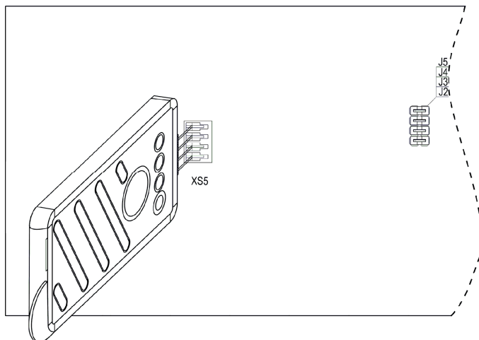
Рис. 1 Подключение USB-программатора к плате ППКОП «ЦИРКОН-3...-8»
