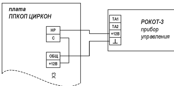
Рис. 8 Подключение прибора речевого оповещения «РОКОТ-3»
