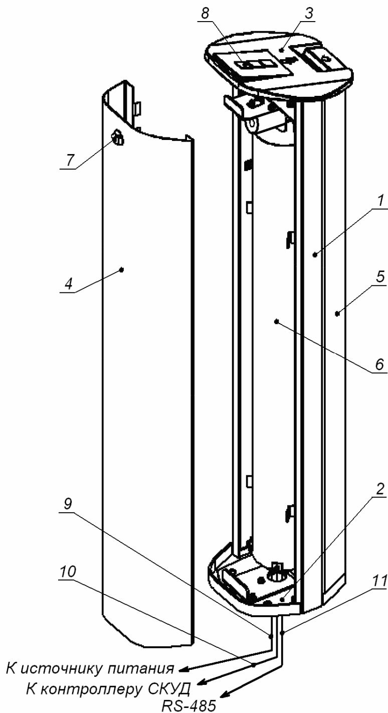
Рисунок 2 Устройство картоприемника:
