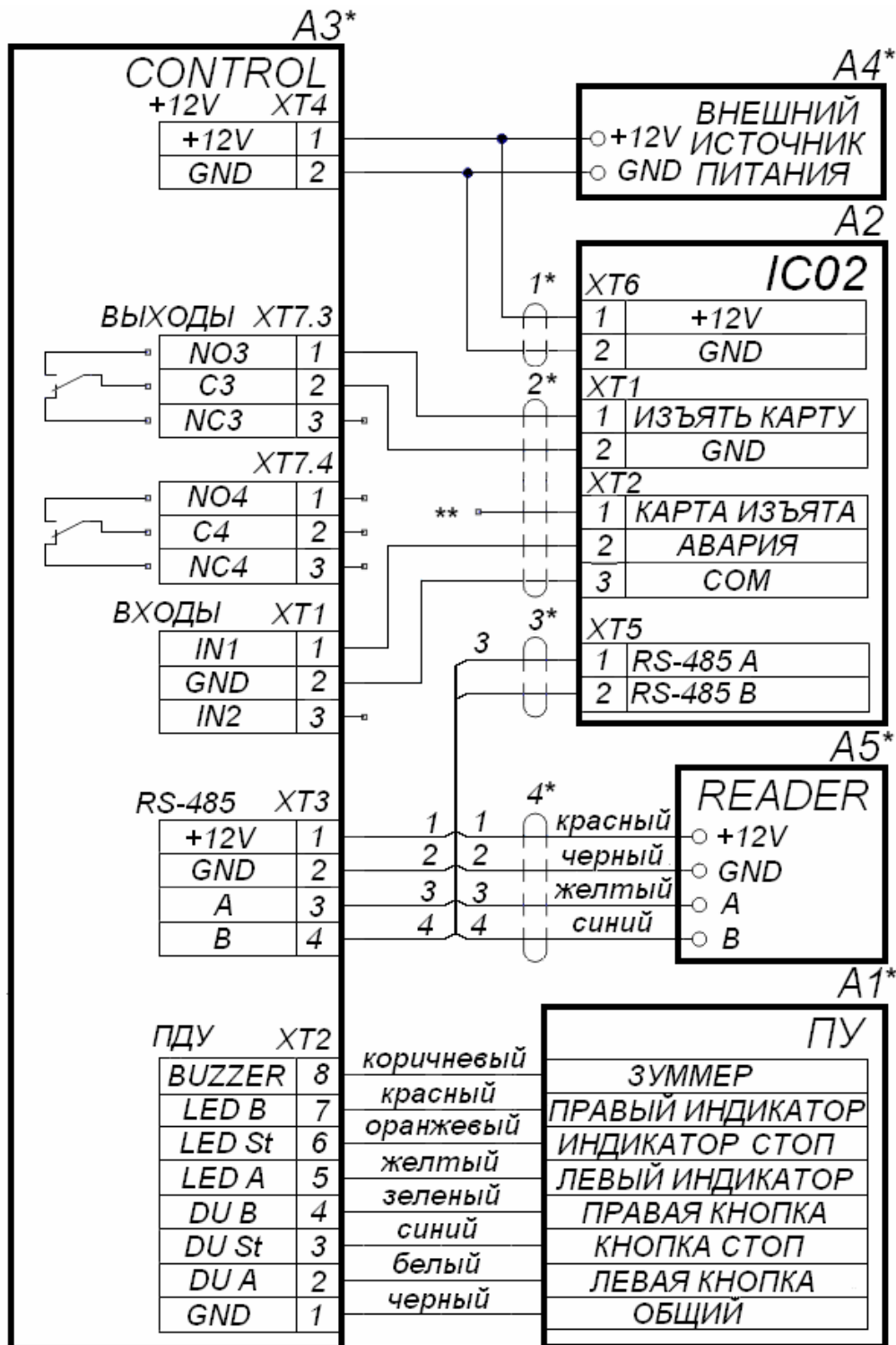
Рисунок 7 Схема подключения картоприемника к контроллеру PERCo-CT/L04 (перечень элементов схемы приведен в таблице 2)
