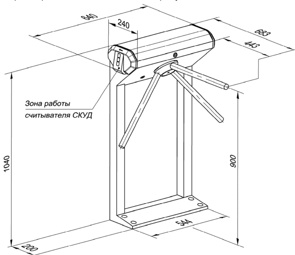
Рисунок 5 Габаритные размеры ЭП
