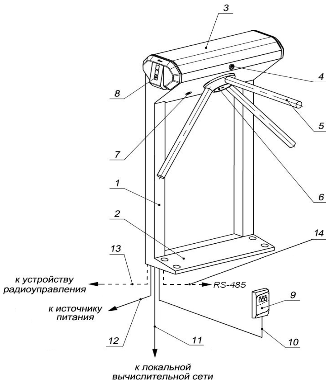
Рисунок 1 Устройство ЭП:
