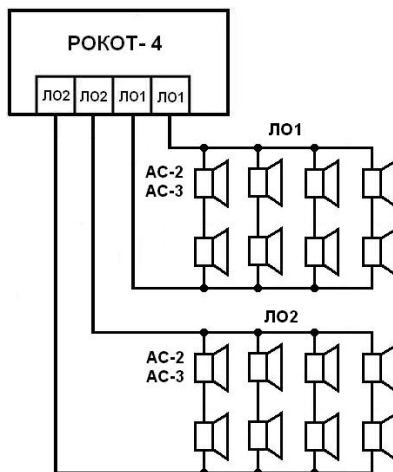
Рис. 3 Схема подключения акустических систем «АС-2-1», «АС-3-1», «АС-3-3»
