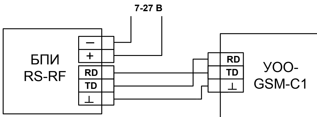
2) Подключение БПИ RS-RF к YOO-GSM-C1
