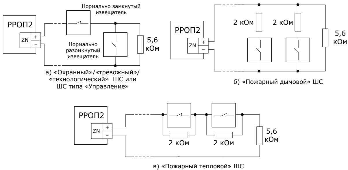
Рисунок В.4 – Подключение в ШС PPOП2 извещателей с выходом типа "сухой контакт"
