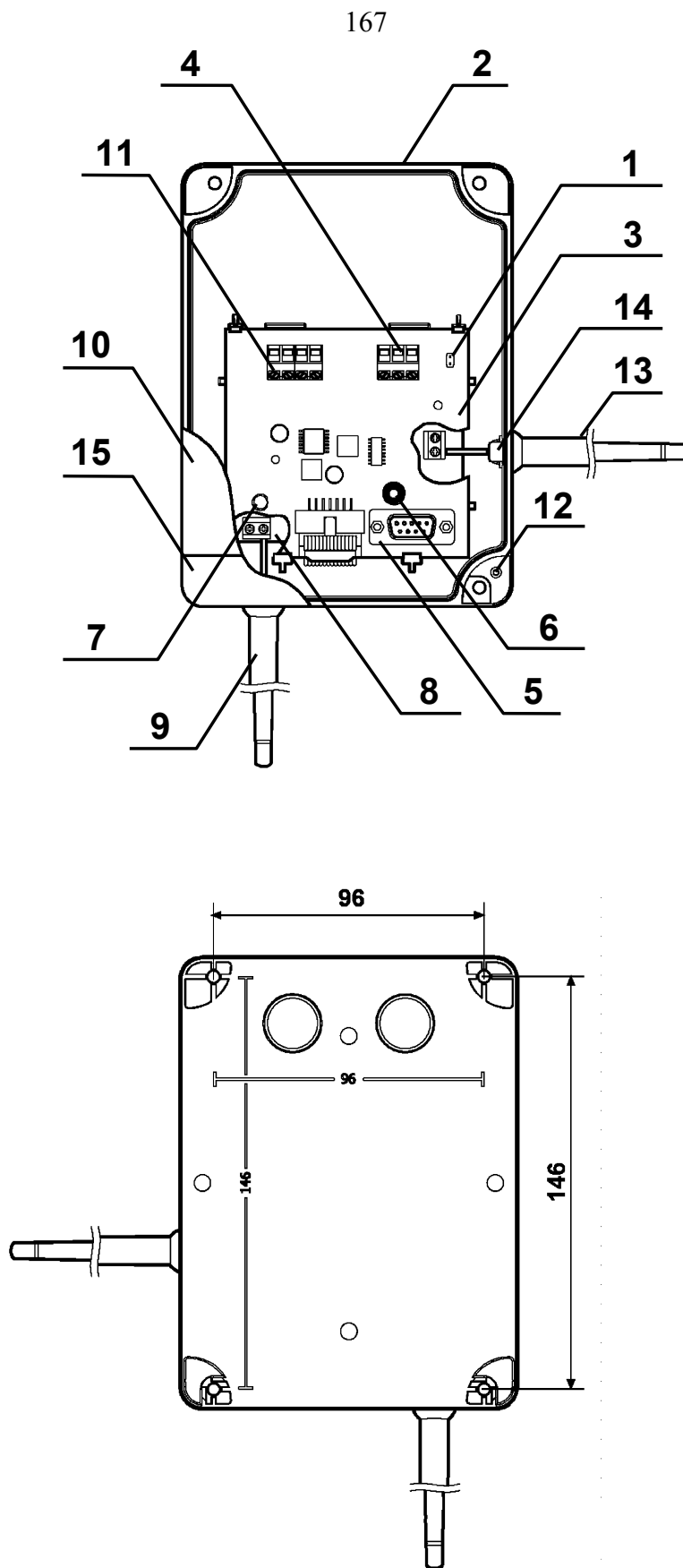
Рисунок Б.4 – Внешний вид РРОП-М исп. У
