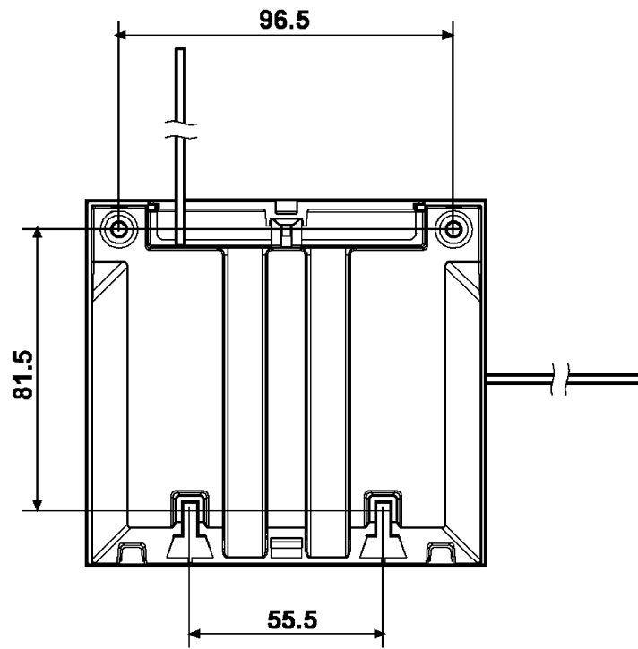
Рисунок Б.3 – Внешний вид РРОП-М
