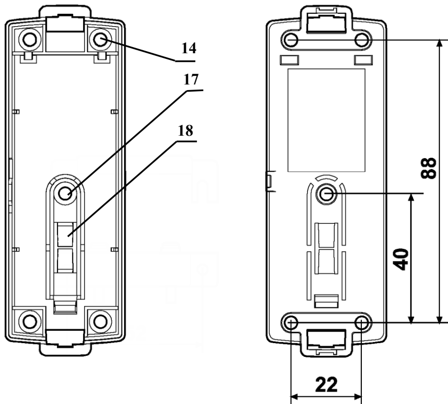
Рисунок Б.31 – Внешний вид технологического детектора "Градус-Р"
