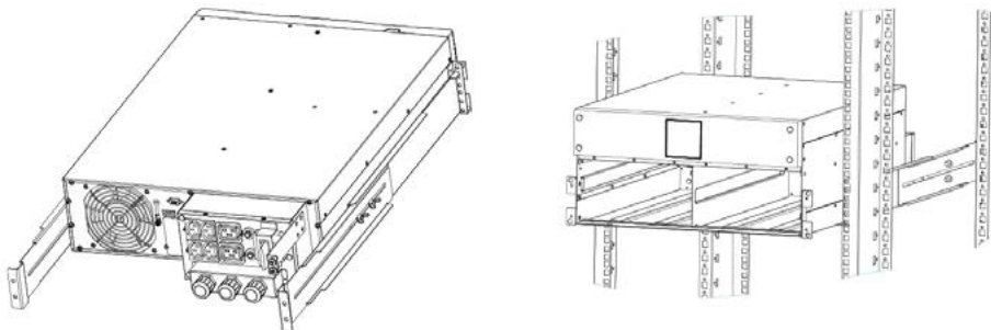
Рисунок 3-12. Установка выдвжных рельсов
