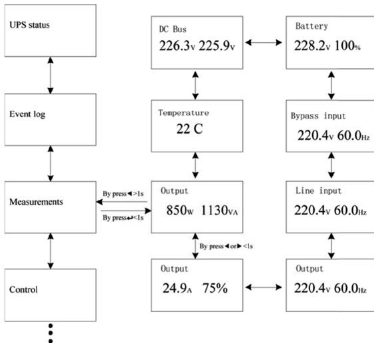
Рисунок 5-16. Меню измерений
