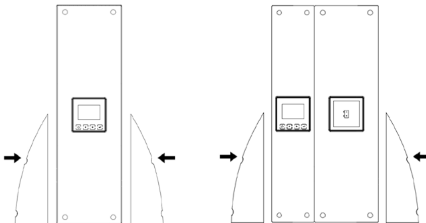
Рисунок 3-17. Вертикальная установка
