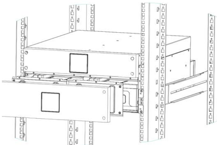
Рисунок 3-13. Монтаж изделия
