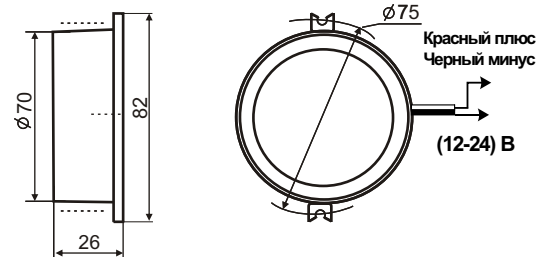
Рис.1. Габаритные и установочные размеры.
