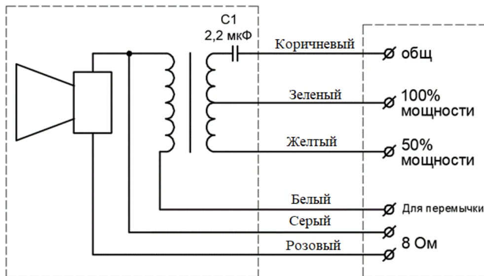
Рисунок 2 – Схема подключения оповещателя
