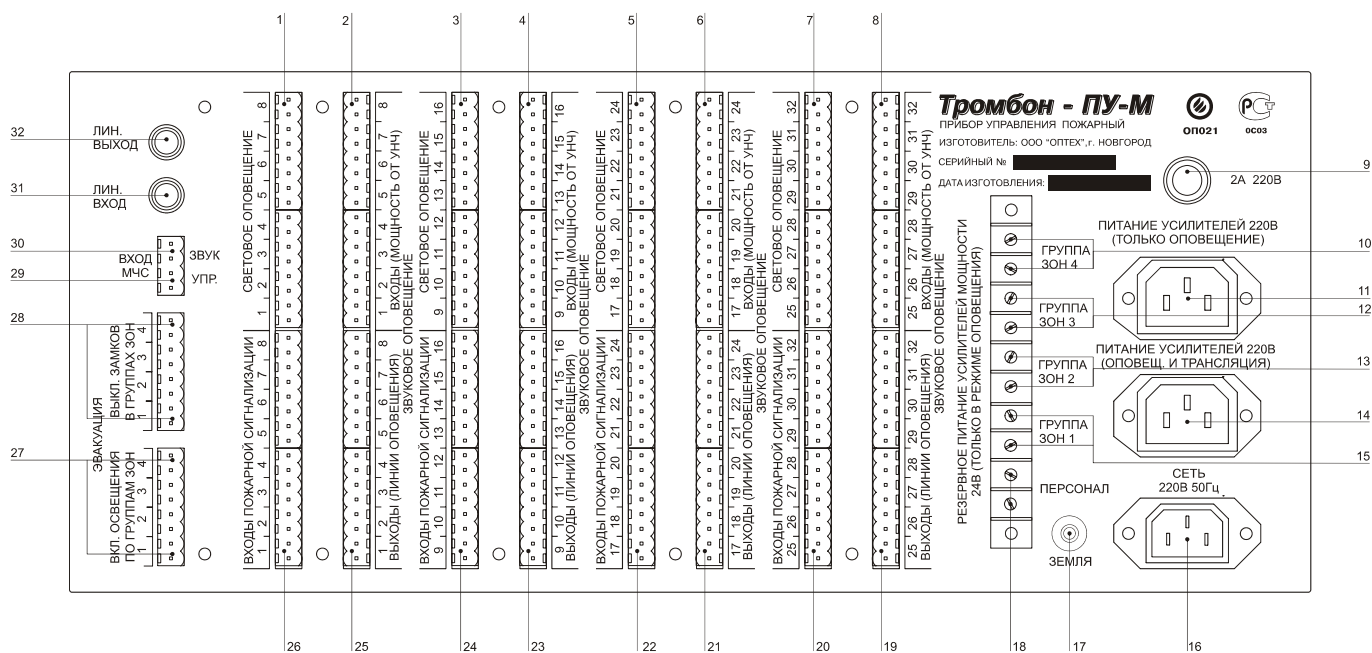
Рис. 2. Прибор управления, вид со стороны задней стенки.
