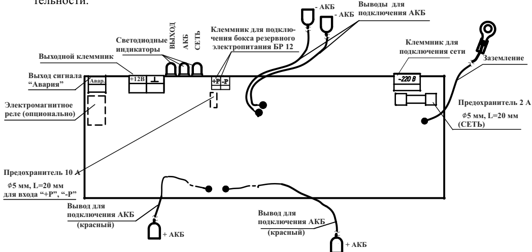
Рисунок 1 – Плата источника
