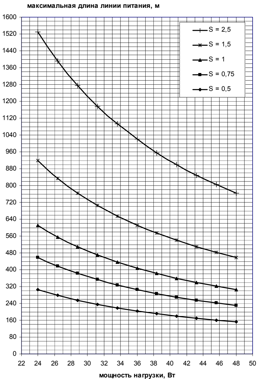
Рис. 3 Максимальная длина линии питания преобразователя при работе с ИБП 60 В
