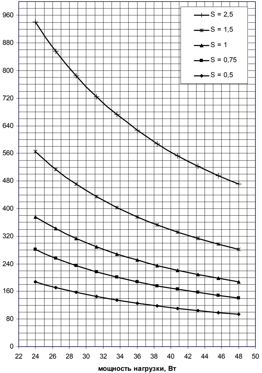
Рис. 2 Максимальная длина линии питания преобразователя при работе с ИБП 48 В
