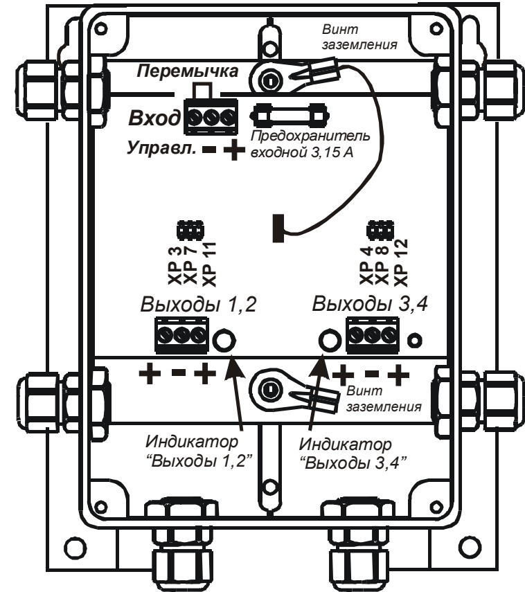
Рис 1. Элементы коммутации, индикации, управления и защиты
