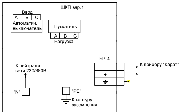
Рис. 1 Схема электрическая подключения шкафов ШКП-04 вар.1
