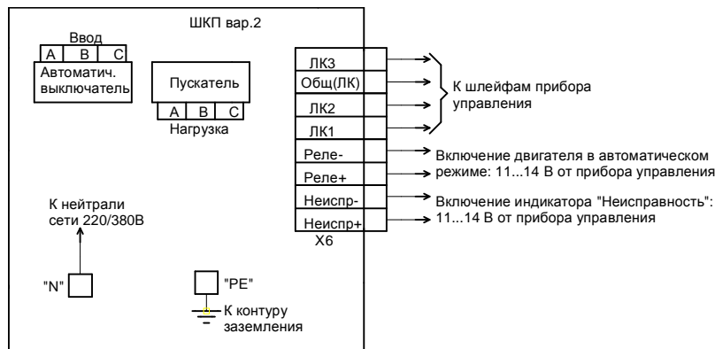
Рис. 2 Схема электрическая подключения шкафов ШКП-04 вар. 2
