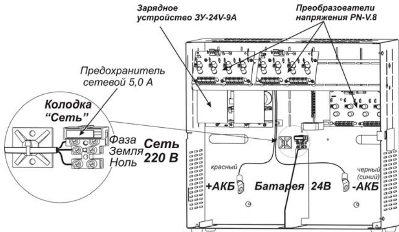
Рис.1 Внешний вид блока с открытой крышкой (базовый вариант)
