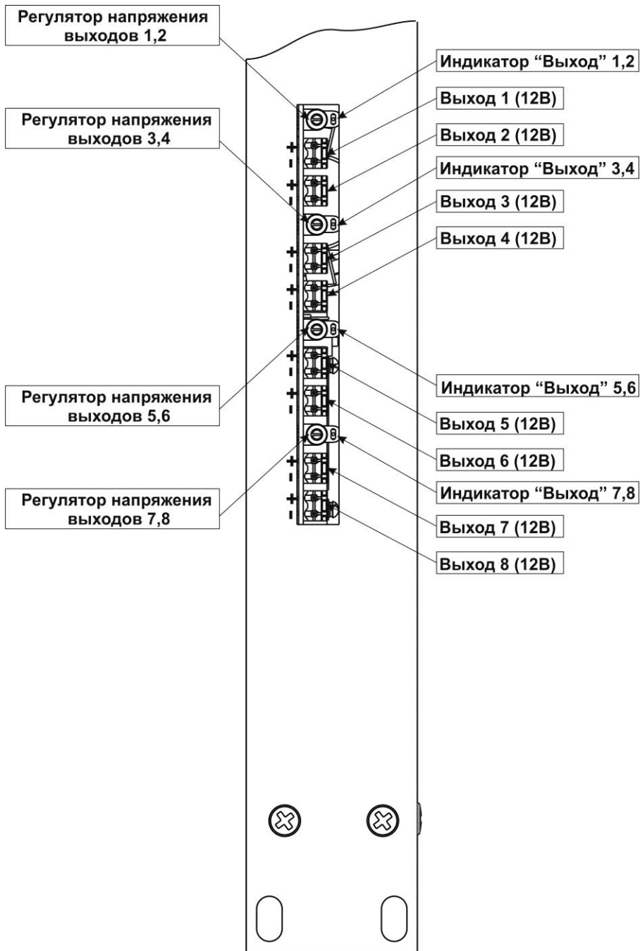
Рис. 2 Схема PN-V.8
