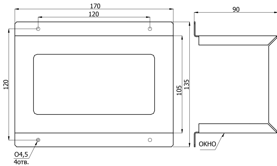
Рис. 1 Общий вид кожуха
