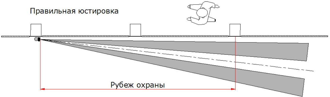
Рис.1.9 Юстировка извещателя на зону обнаружения.
