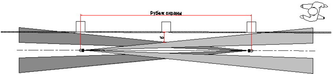
Рис.1.9 Юстировка извещателя на зону обнаружения.
