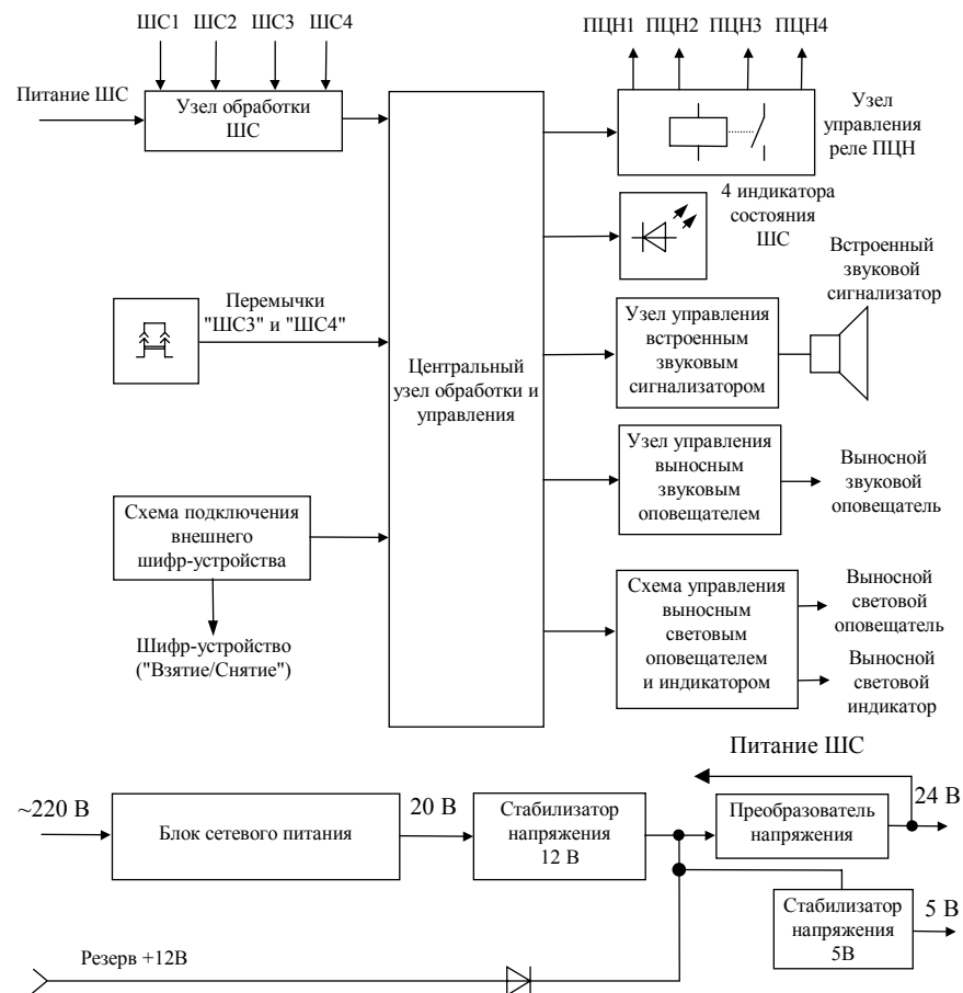
Приложение Б Схема электрическая функциональная прибора (обязательное)
