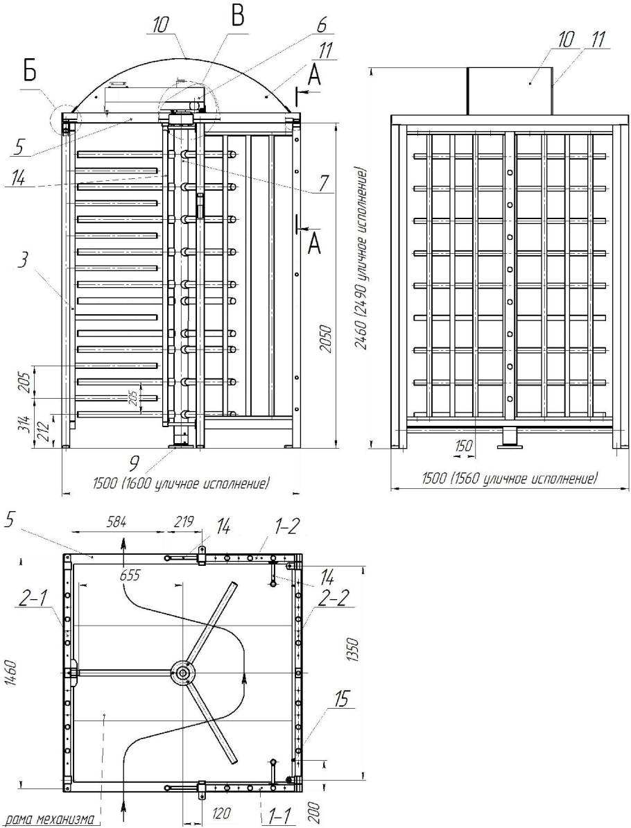
Турникет «Ростов-Дон ПР1Ш/ЗМ» в режиме шлюза
