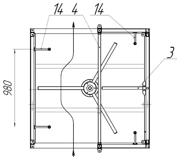
Турникет «Ростов-Дон ПР1Ш/3М» в режиме турникета (остальное см. Приложение 1.1)
