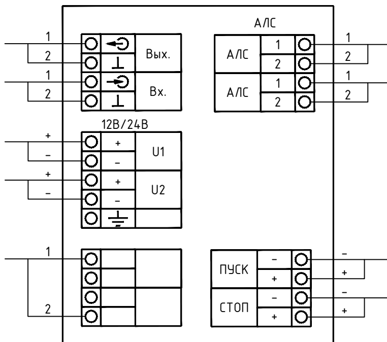
Типовая схема подключения "МРО-2М прот. R3" (xAy.z)
