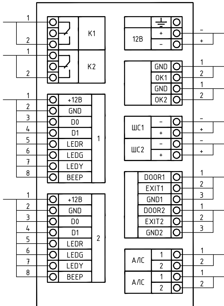
Типовая схема подключения "МКД-2 прот. R3" (xAy.z)
