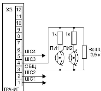
Рис. 6 Подключение токопотребляющих пожарных извещателей
