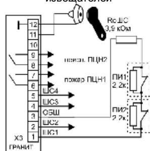
Рис. 5 Подключение пассивных пожарных извещателей
