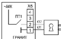
Рис. 4 Подключение электромагнитного замка
