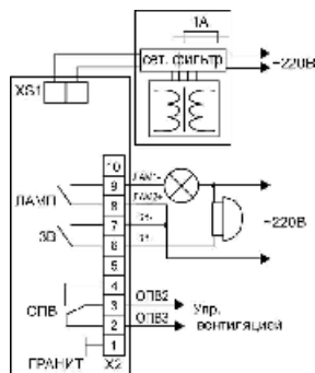
Рис. 2 Подключение сети, оповещателей с питанием от сети и управления вентиляцией
