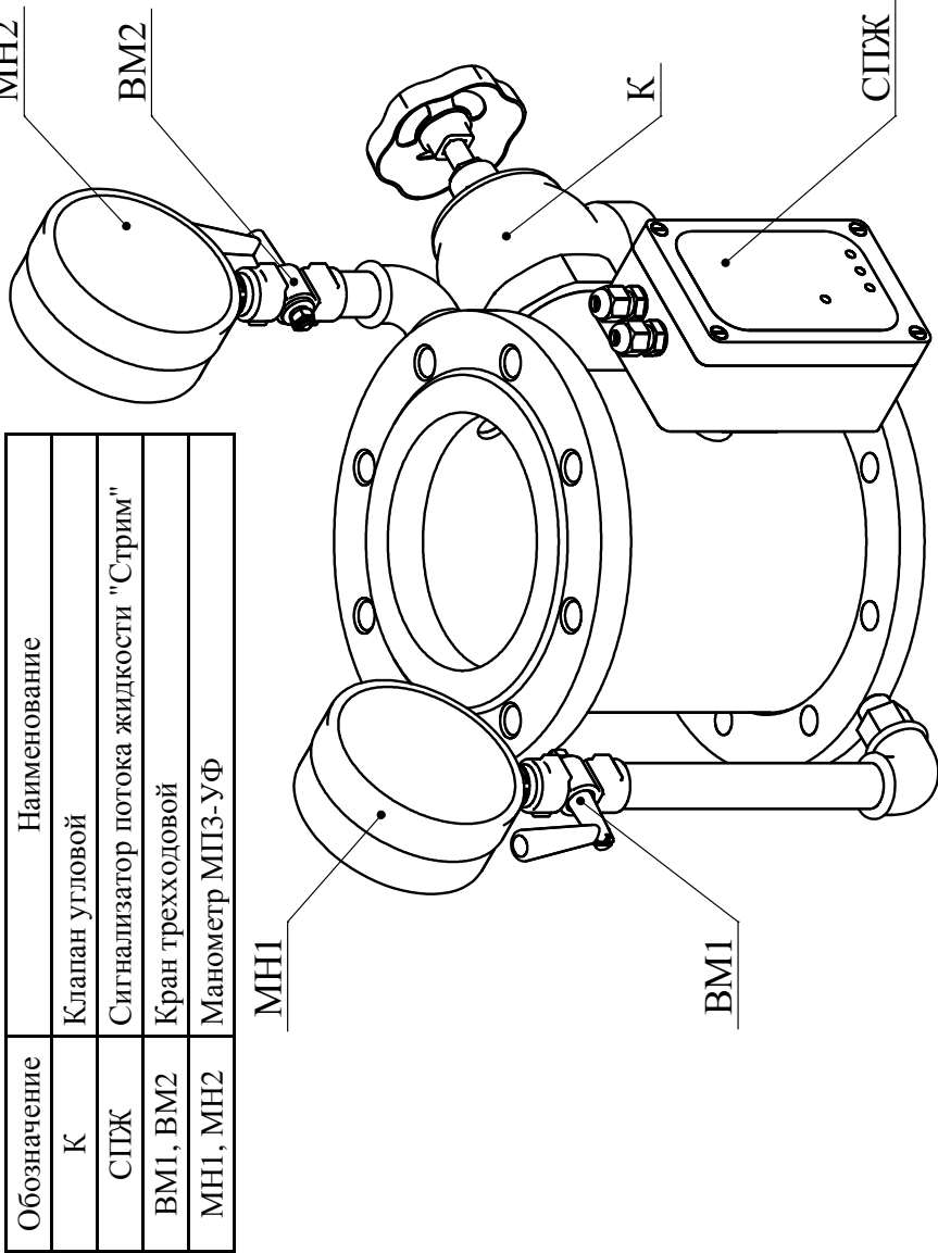
Рисунок 2 - Узел управления спринклерный водозаполненный "Шалтан"
