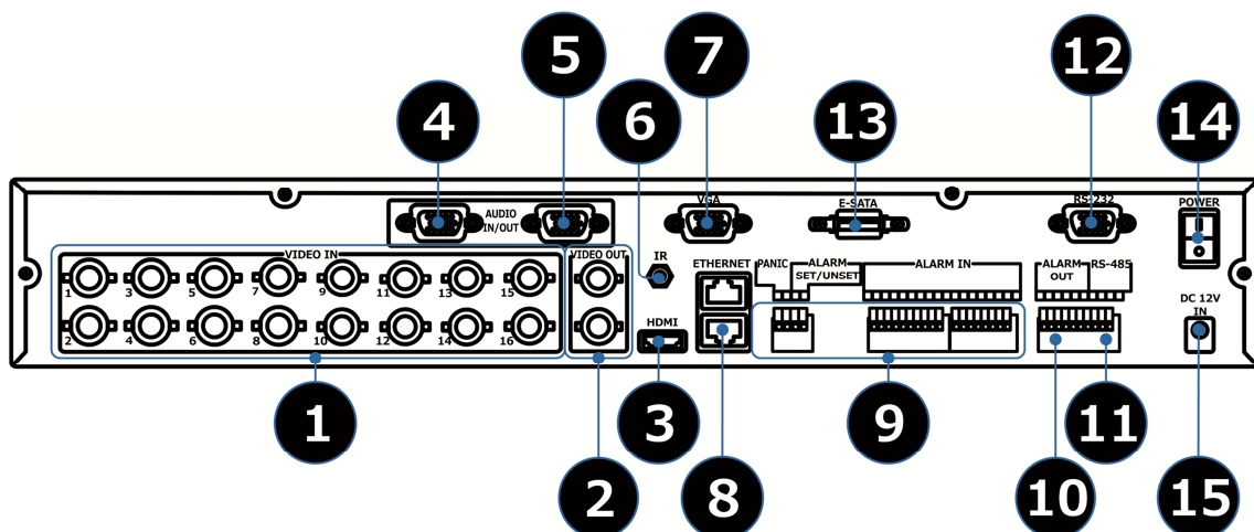
HQ-9716, вид сзади (16 каналов).
