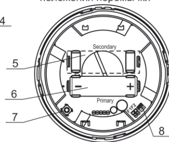
Электронный блок Вид снизу Элемент питания установлен
