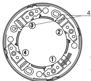
База Электронный блок снят
